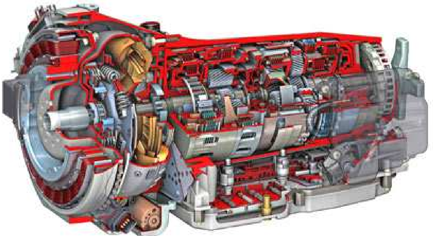
Modifiziertes Getriebe mit E-Motor
