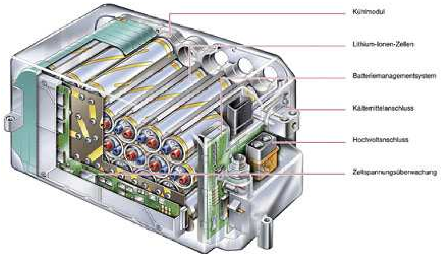
Bild 1: Lithium-Ionen-Hochvoltbatterie
